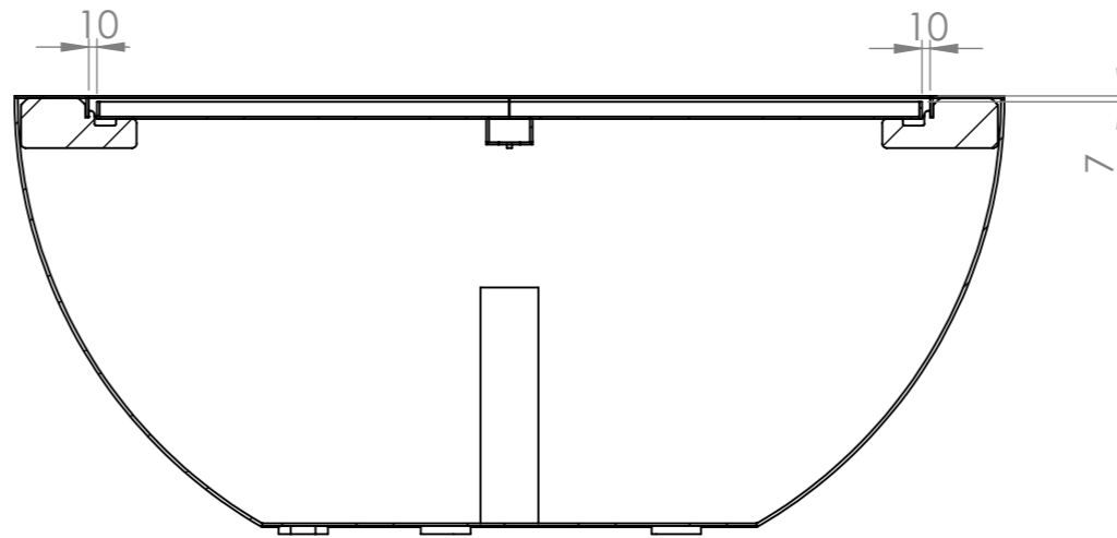
SECTION D-D
